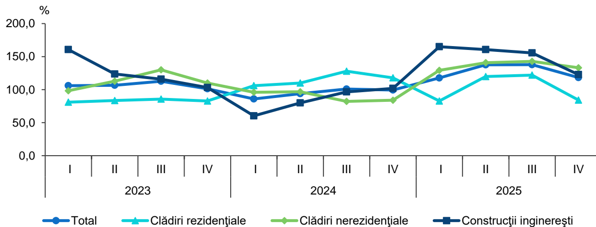
Figura 10.2. Indicii volumului lucrărilor de construcții executate, pe obiecte de construcții, în anii 2023-2025 (pe trimestre), în % față de perioada corespunzătoare a anului precedent
